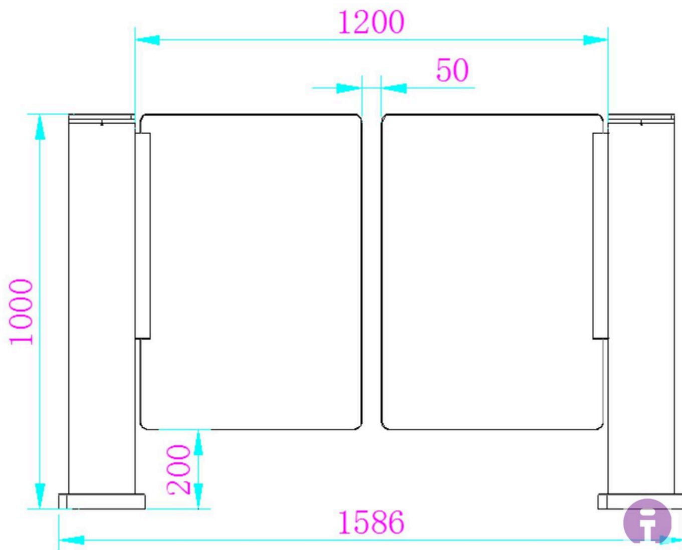
VISTA FRONTALE, DOPPIA ANTA
