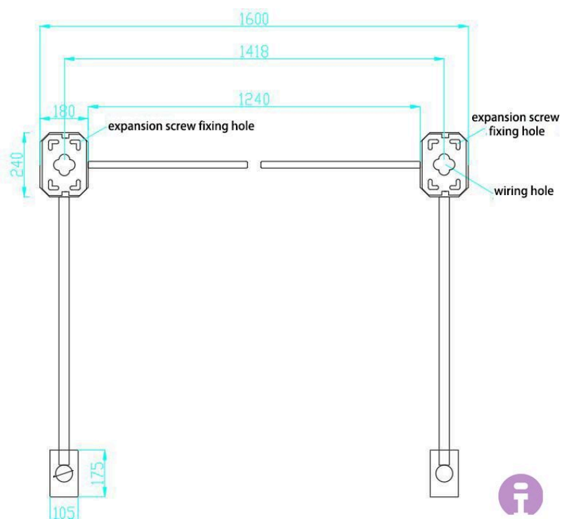
PIANTA CON INTERASSE DI FISSAGGIO
