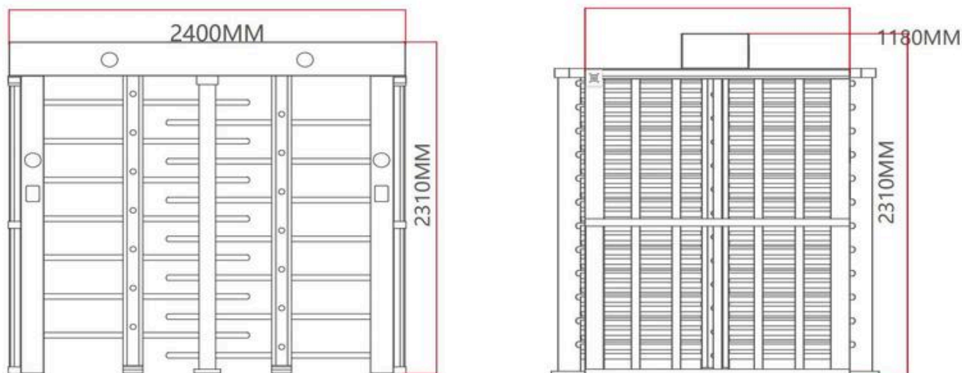
VISTA FRONTALE E LATERALE
